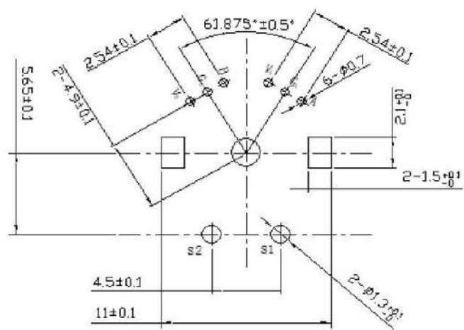
PCB孔位尺寸图 PCB hole size diagram
