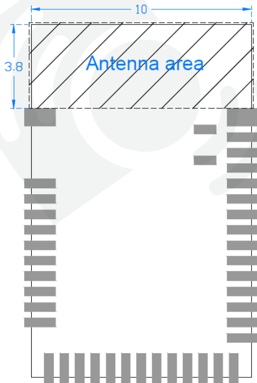
Antenna area
