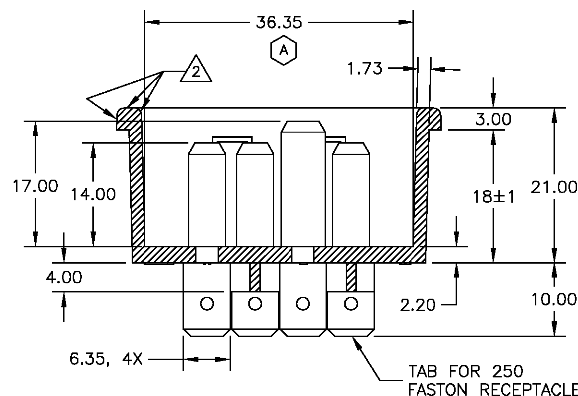
SECTION A-A
