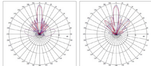
Detachable 14x16 4.9-5.85 GHz H-Plane E-Plane
