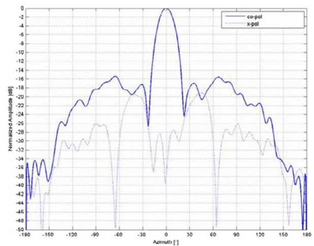
5150-5850 MHz
