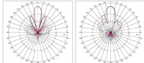
Detachable 14x16 2.4-2.7 GHz H-Plane E-Plane
