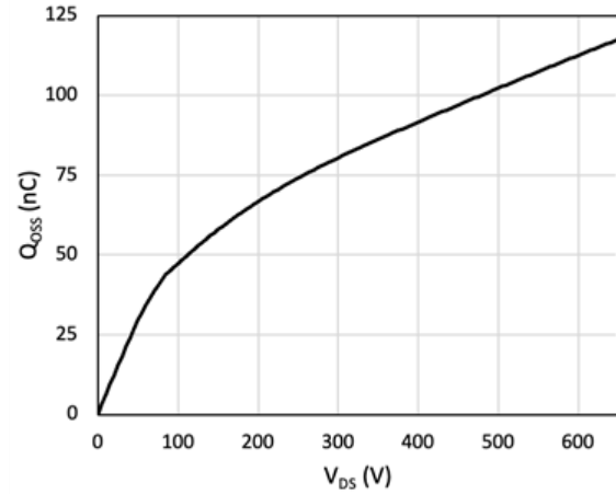
Fig. 10. Q_{OSS} vs. V_{DS}
