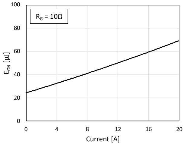
Fig. 15. E_{ON} vs. I_{DS} , T_{JUNC} = 25\text{ °C}
