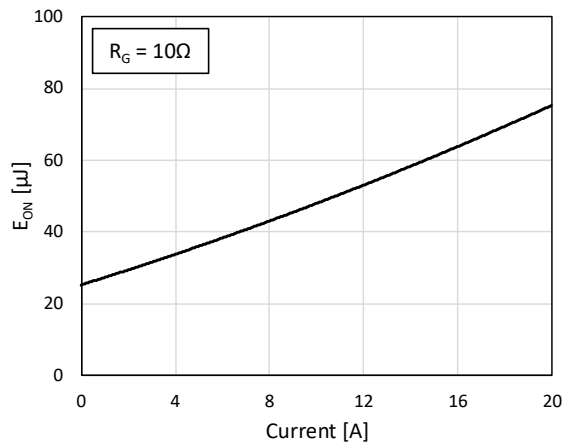
Fig. 17. E_{ON} vs. I_{DS} , T_{JUNC} = 125\text{ °C}
