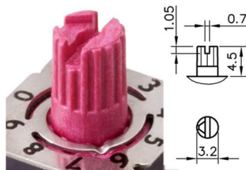
Spindle
