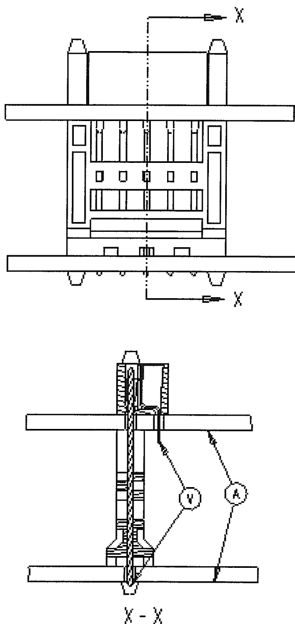
Fig. 3 ローレベル総合抵抗測定
