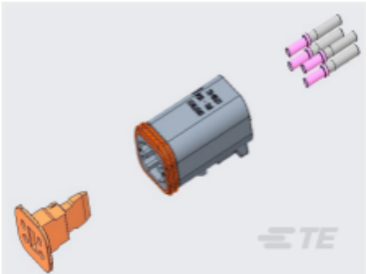
TE Part #DT06-4S-COMplete DT06-4S CON AND WEG
