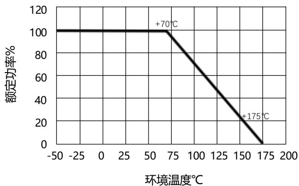
操作温度范围-50~+175℃，电阻温度达到70℃时降功率示意图
