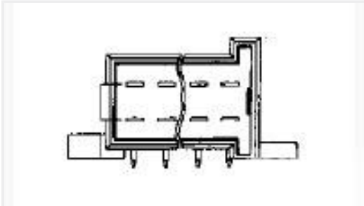
TE Part #828801-2 2X 3P MESSERLEI 3,0
