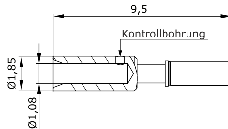
Hauptabmessungen Kontaktbuchse
