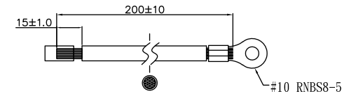
STW 8AWG GREEN (1PC)
